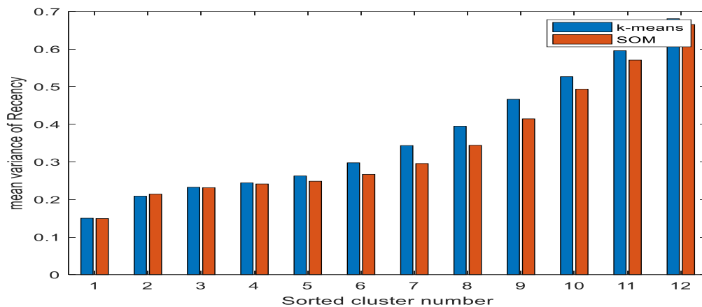
نمودار ۱- میانگین انحراف معیار مقدار R داده‌های درون خوشه
