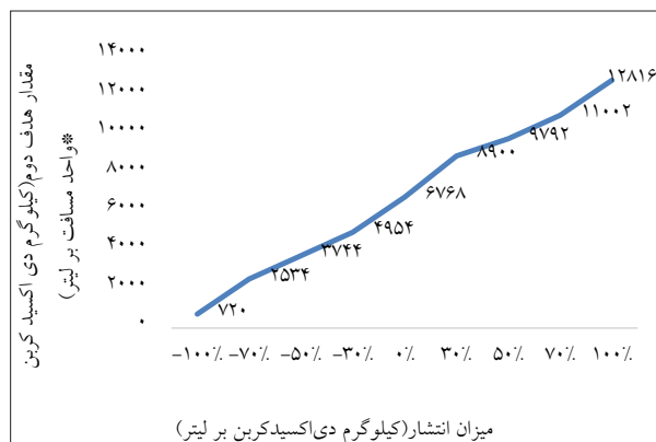
نمودار ۷- تحلیل حساسیت میزان انتشار دی اکسید کربن وسیله نقلیه مرکز توزیع با استفاده از روش اپسیلون- محدودیت برای تابع هدف دوم
