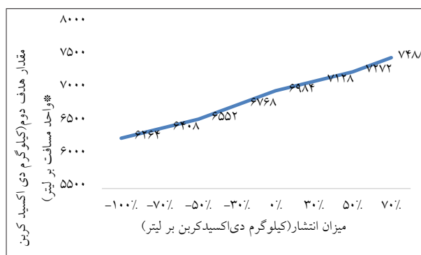
نمودار ۸- اثر تغییر مقدار انتشار دی اکسید کربن وسیله نقلیه مرکز باز یافت برای تابع هدف دوم
